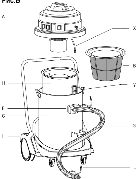
(ВНУТРЕННИЙ БАК)
